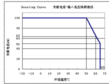
2、负载电流—环境温度降额曲线:
